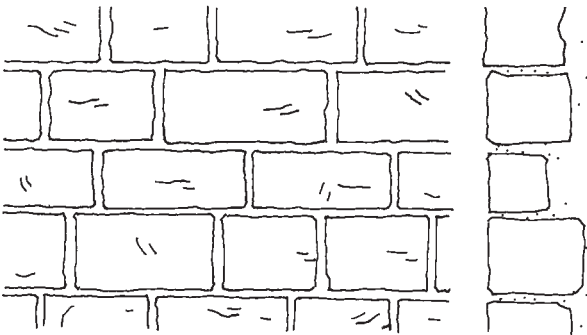
Unregelmässiges Schichtenmauerwerk
