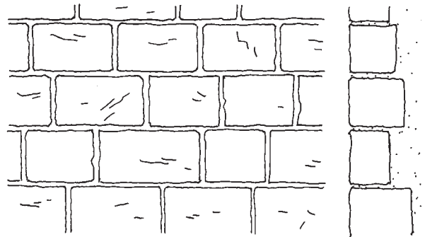
Regelmässiges Schichtenmauerwerk
