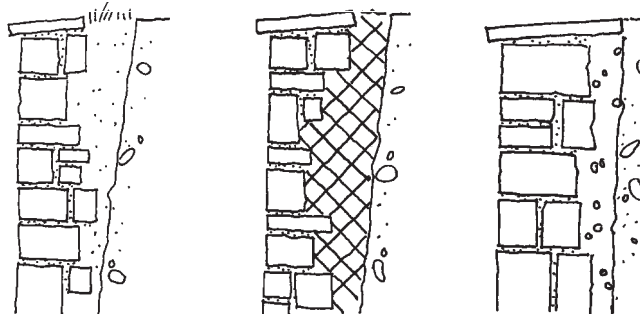
weich hinterfüllt
